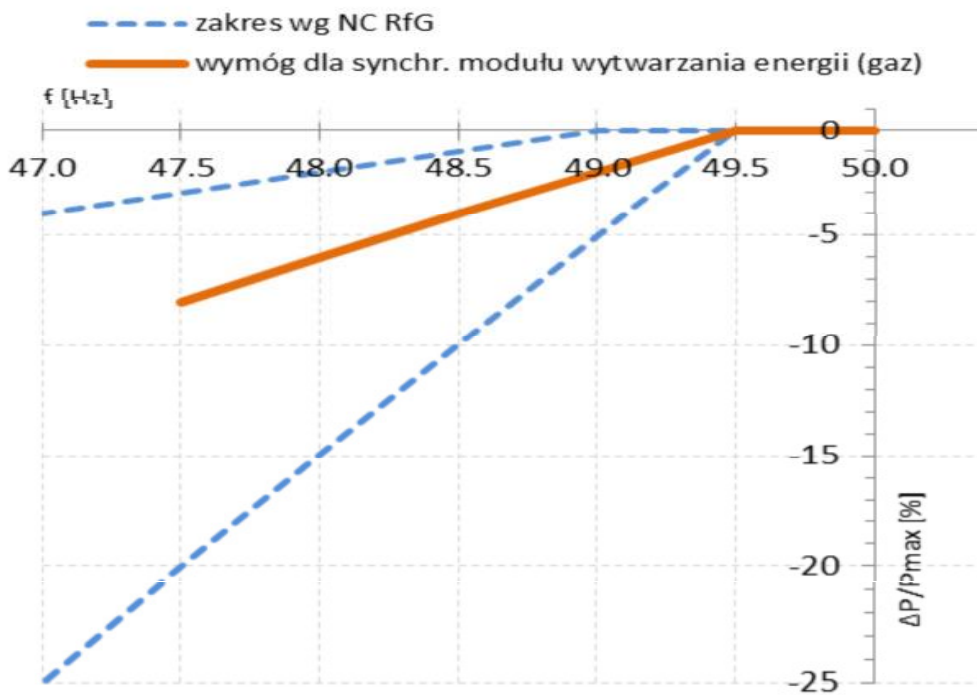
Rys. 3 Maksymalny spadek zdolności do generacji mocy przy spadku częstotliwości dla synchronicznych modułów wytwarzania energii typu blok gazowy lub gazowo-parowy
