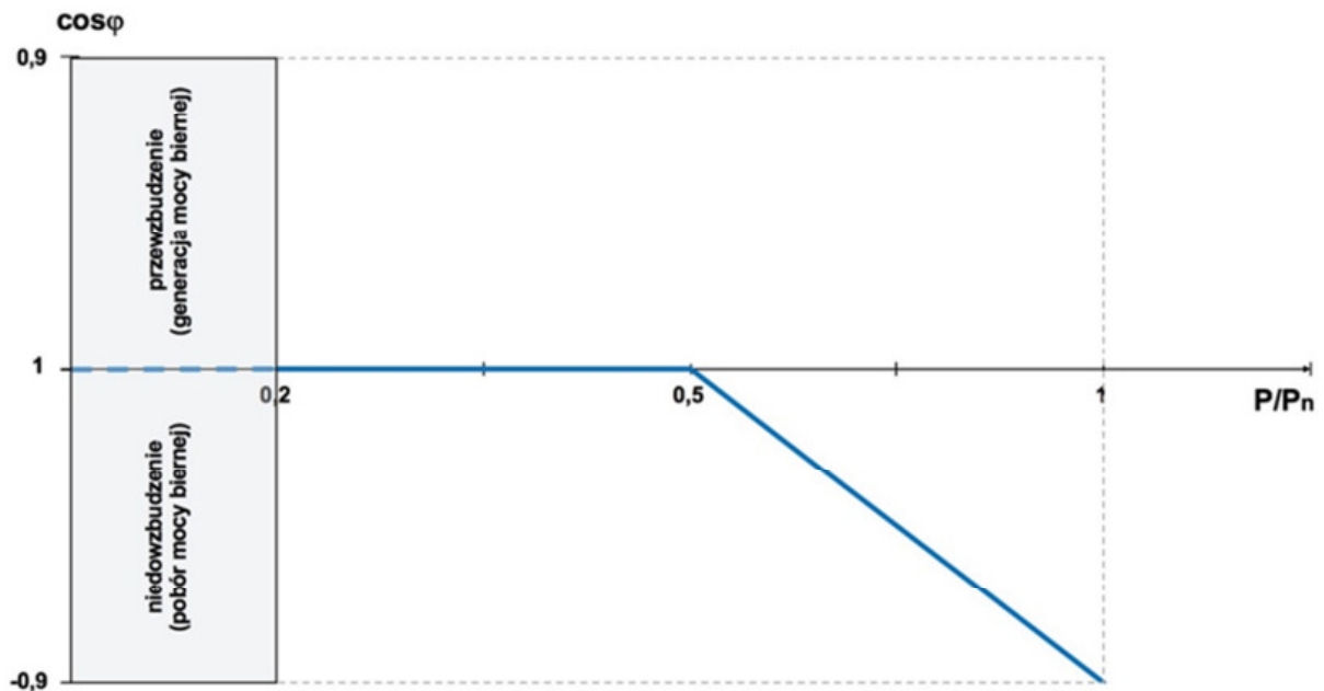
Rys. 5. Charakterystyka sterowania współczynnikiem mocy \cos \phi w funkcji generowanej mocy czynnej wymagana przez OSD
