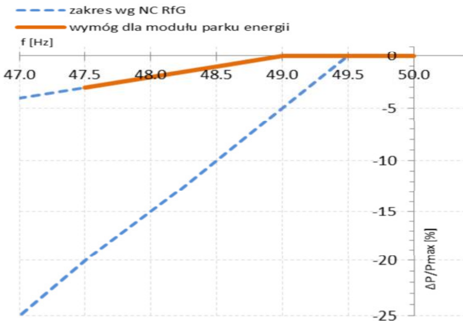
Rys. 4. Maksymalny spadek zdolności do generacji mocy przy spadku częstotliwości dla modułów parku energii
