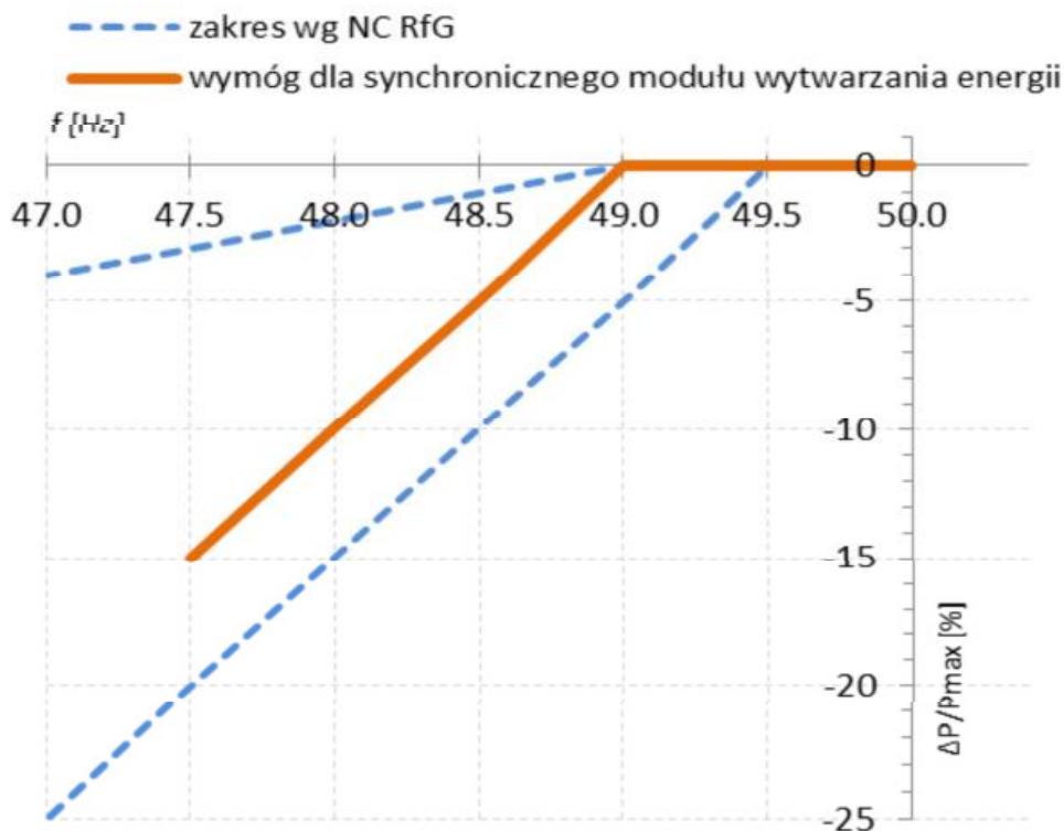
Rys. 2 Maksymalny spadek zdolności do generacji mocy przy spadku częstotliwości dla synchronicznych modułów wytwarzania energii z wyłączeniem bloku gazowego lub gazowo-parowego
